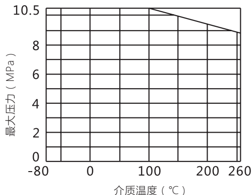
图 8 平衡密封环使用温度、压力范围
