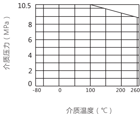
图 7 平衡密封环使用作温度、压力范围
