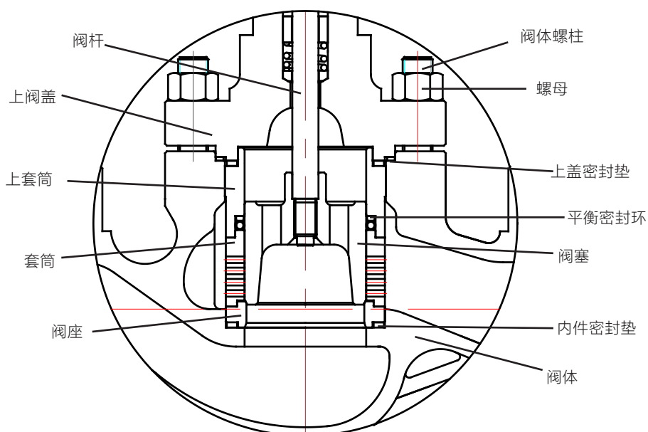
图1 LN8510 阀体组件结构图
