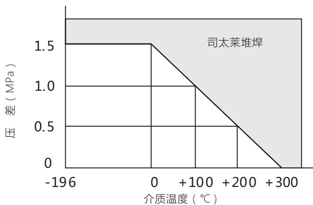
图 6 司太莱堆焊工作温度、压力范围
