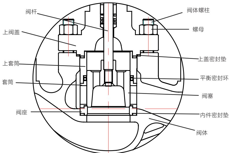
图 1 LN8500 阀体组件结构图
