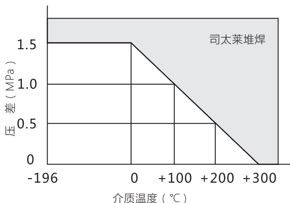
图 7 司太莱堆焊工作温度、压力范围
