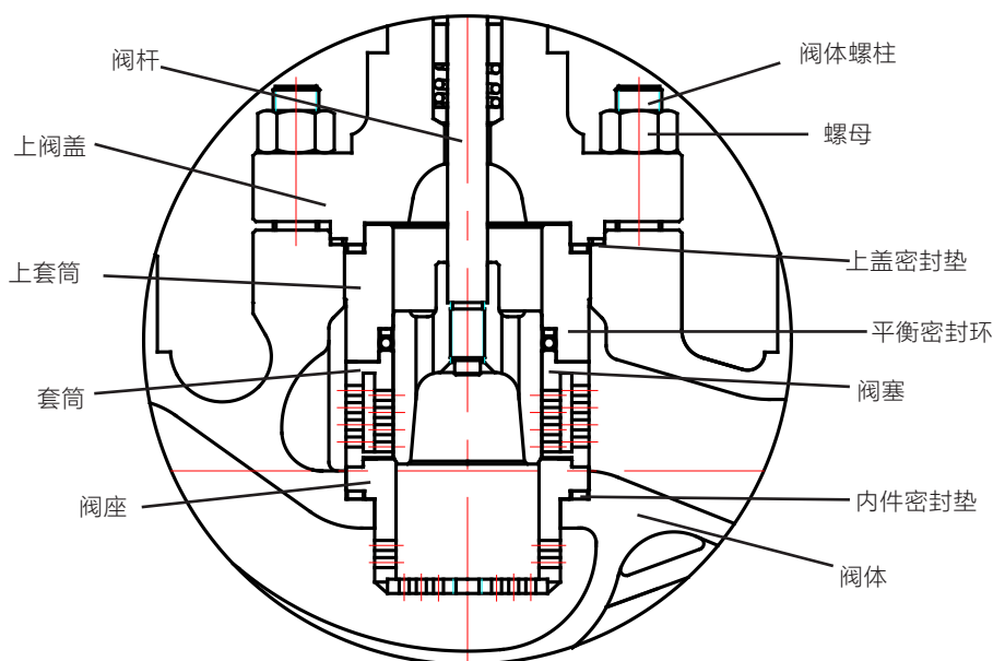
图 1 LN8560 阀体组件结构图
