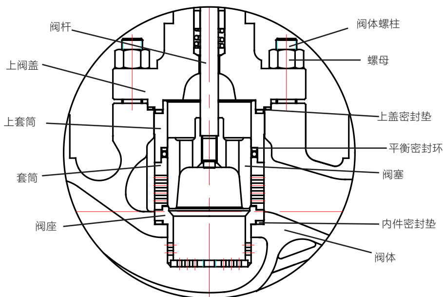
图 1 LN8520 阀体组件结构图
