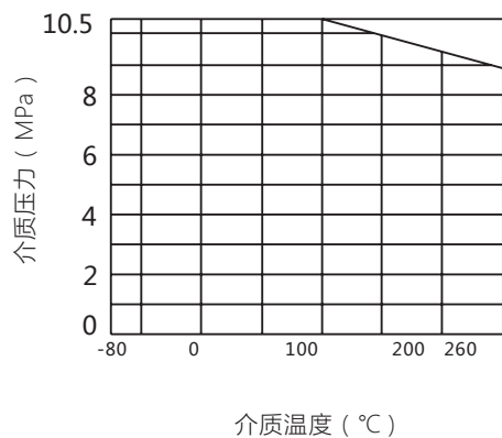
图 7 平衡密封环使用温度、压力范围
