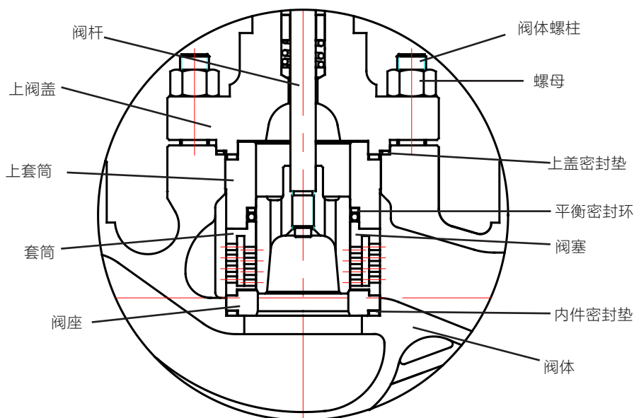
图 1 LN8550 阀体组件结构图
