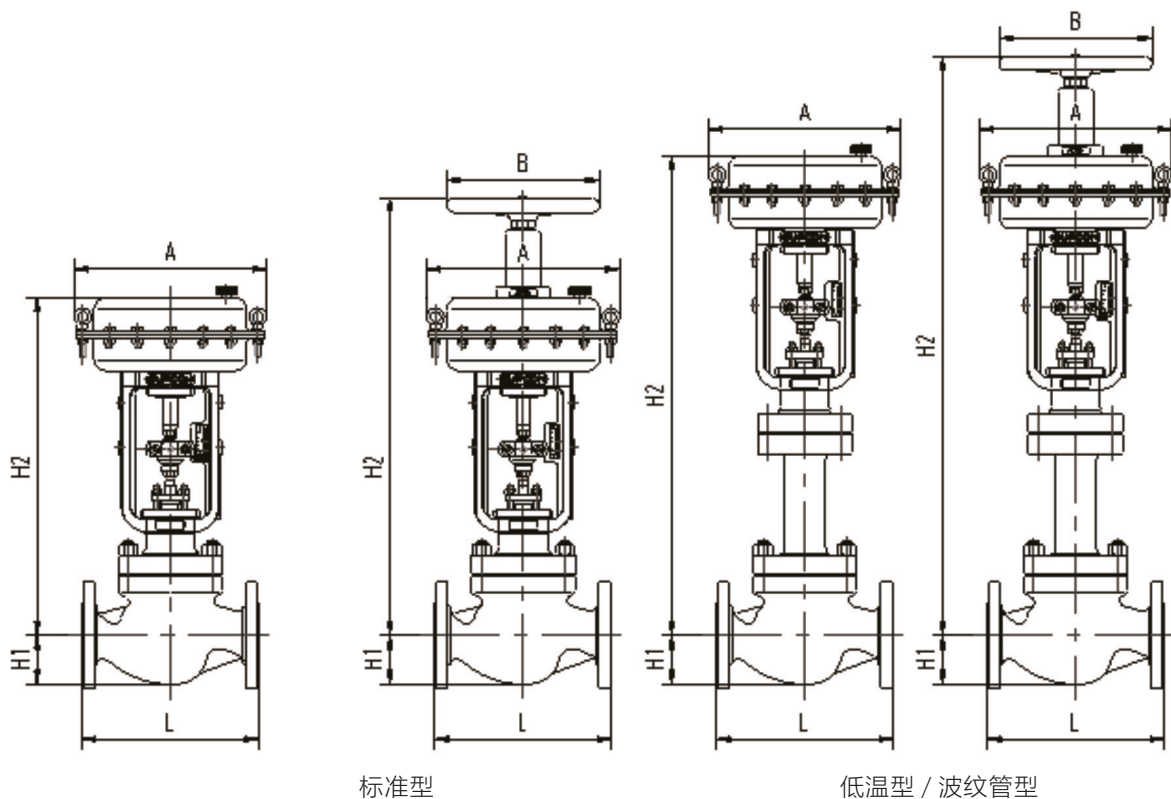
图 9 配 AM8 执行机构、DS8 手轮外型尺寸图
