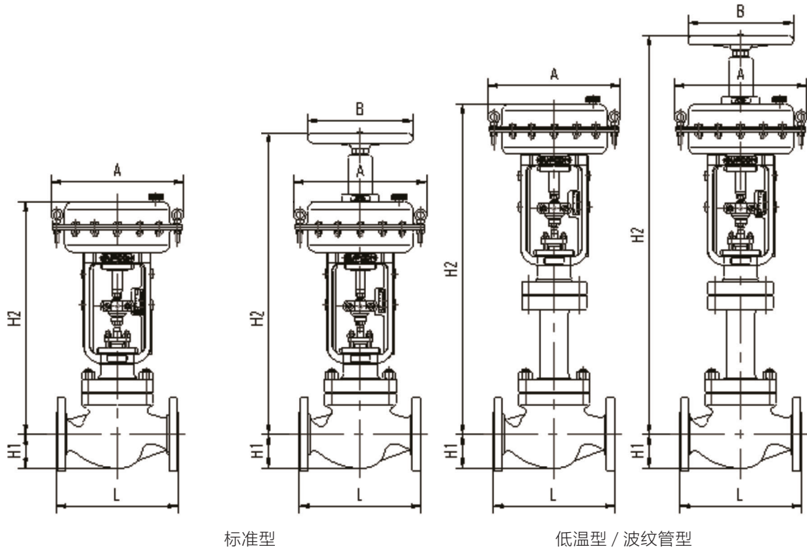
图 8 配 AM8 执行机构、DS8 手轮外型尺寸图
