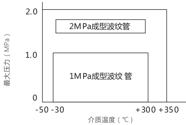
图 6 波纹管上阀盖工作温度、压力范围
