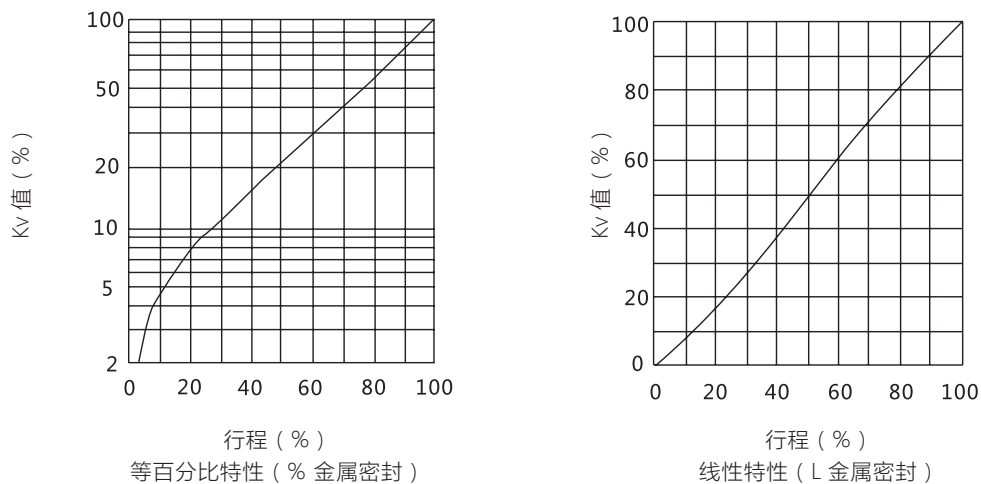
图 3 流量特性曲线 (高特性型)
