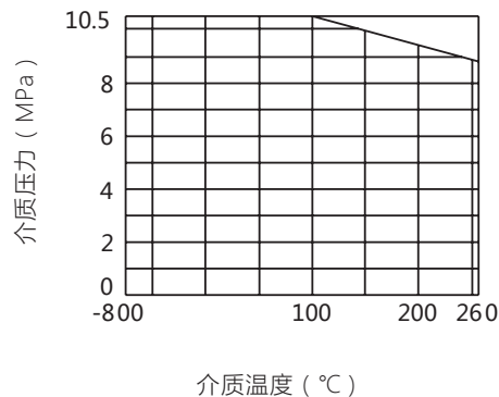
图 7 平衡密封环使用作温度、压力范围
