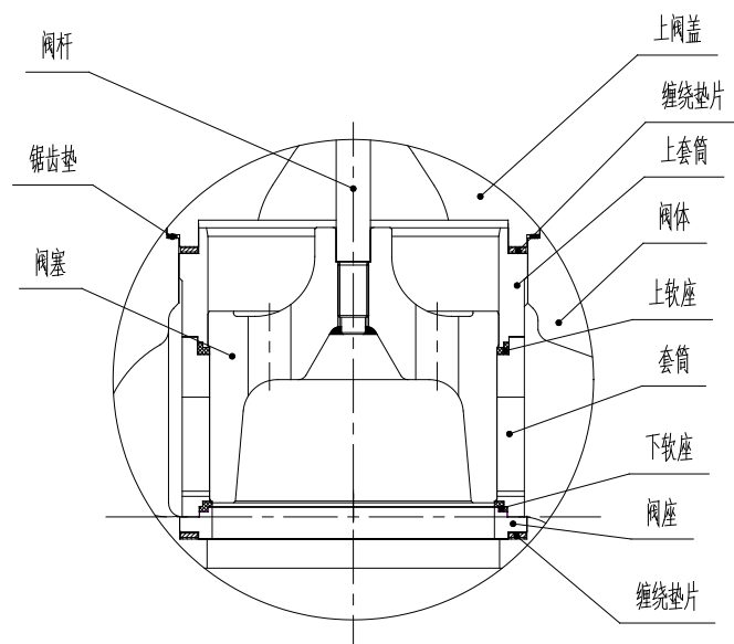
图 1 LN8530 阀体组件结构图
