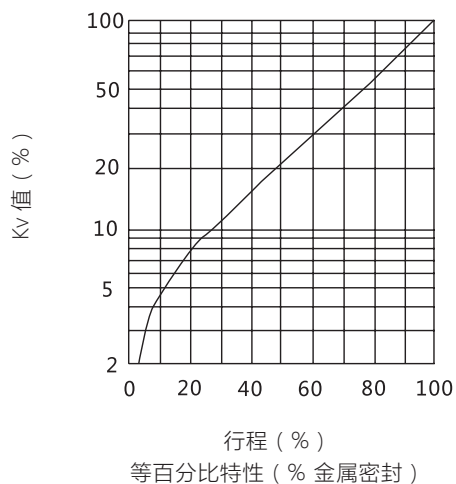
图 3 流量特性曲线 (高特性型)
