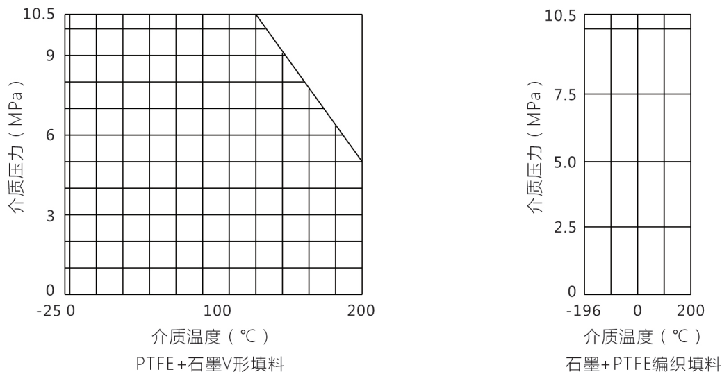
图 5 填料使用温度、压力范围
