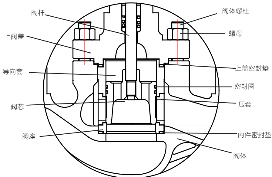
图 1 LN8300 阀体组件结构图
