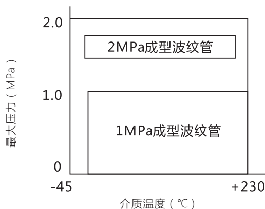
图 8 波纹管上阀盖工作温度、压力范围
