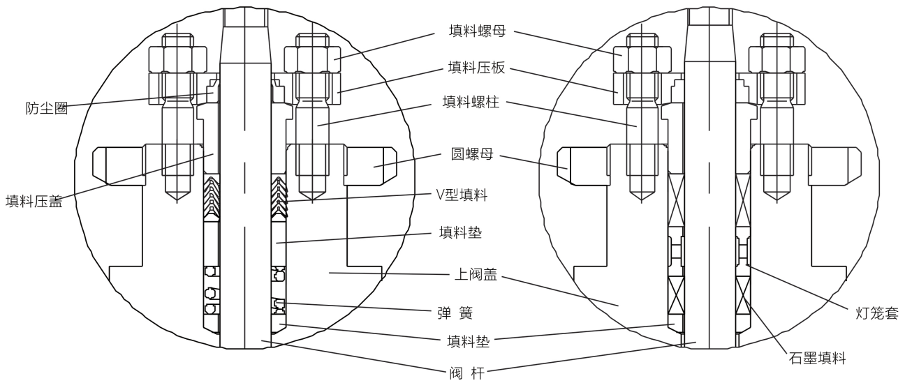
图 4 PTFE+ 石墨 V 形填料
