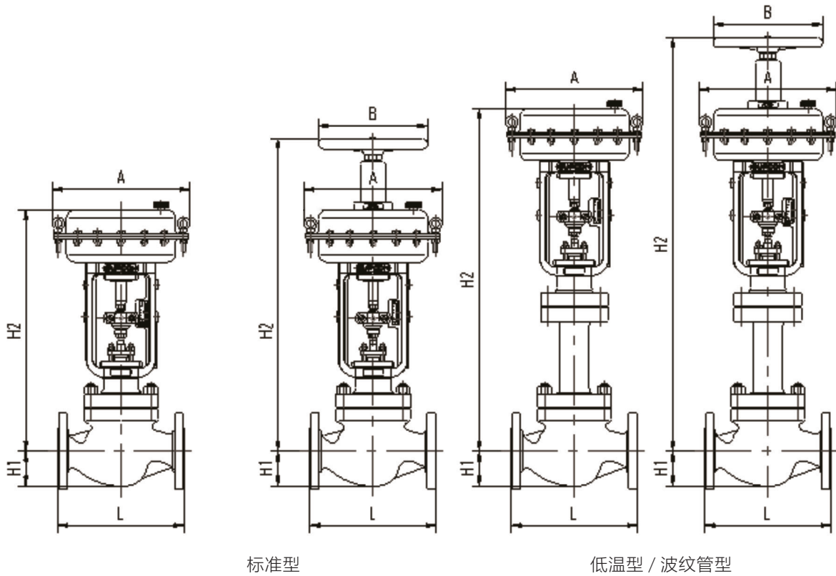
图 8 配 AM8 执行机构、DS8 手轮外型尺寸图
