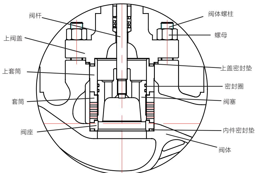
图 1 LN8310 阀体组件结构图
