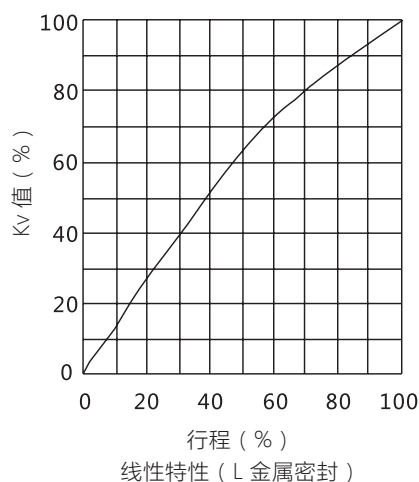
图 2 流量特性曲线 (大容量型)
