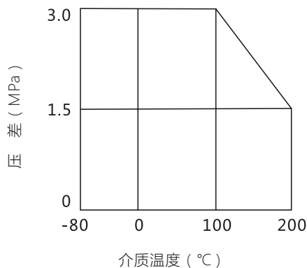
图 9 密封圈使用温度、压力范围
