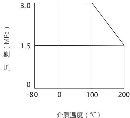
图 7 密封圈使用作温度、压力范围
