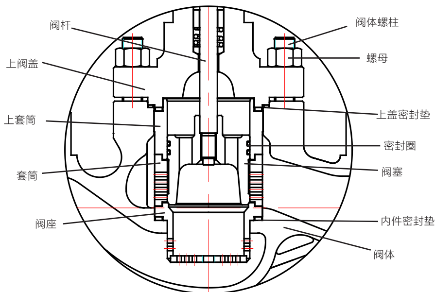
图 1 LN8320 阀体组件结构图
