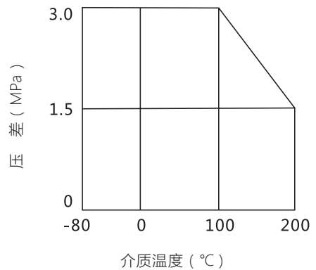
图 7 密封圈使用作温度、压力范围
